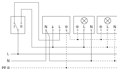
Schaltplan Anschluss über einen Wechselschalter für Dauerlicht- und Automatik-Betrieb
